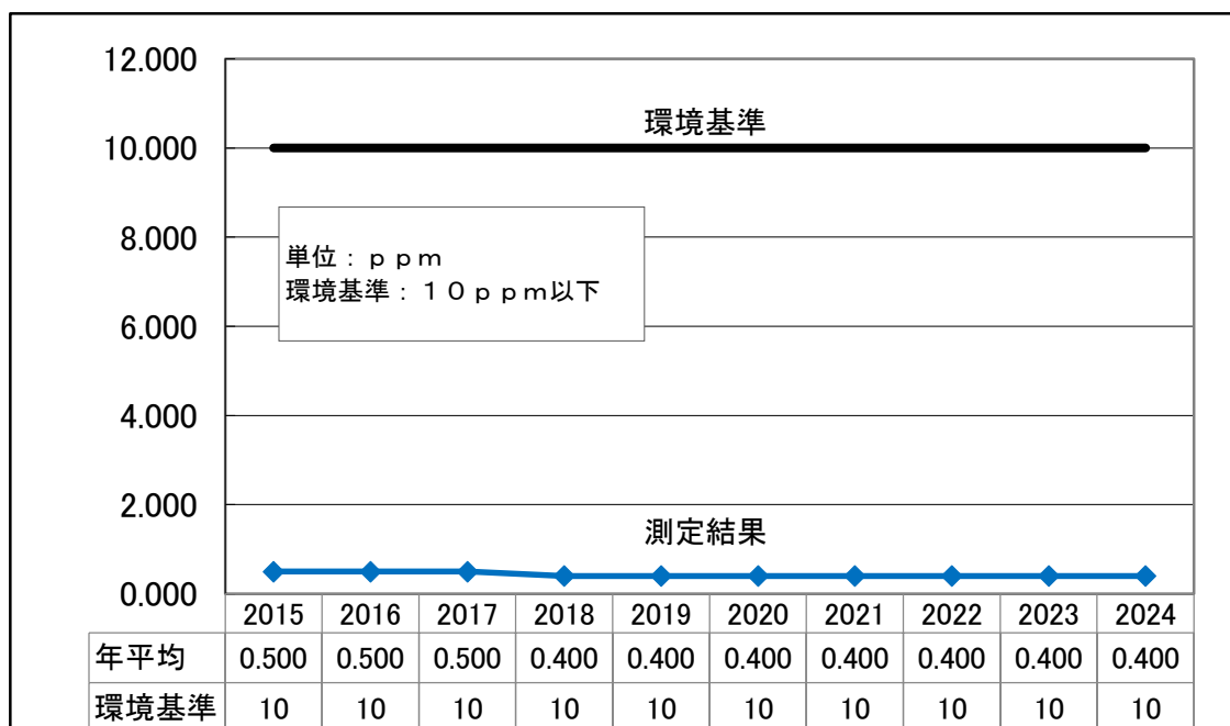
図15 一酸化炭素濃度の測定結果
