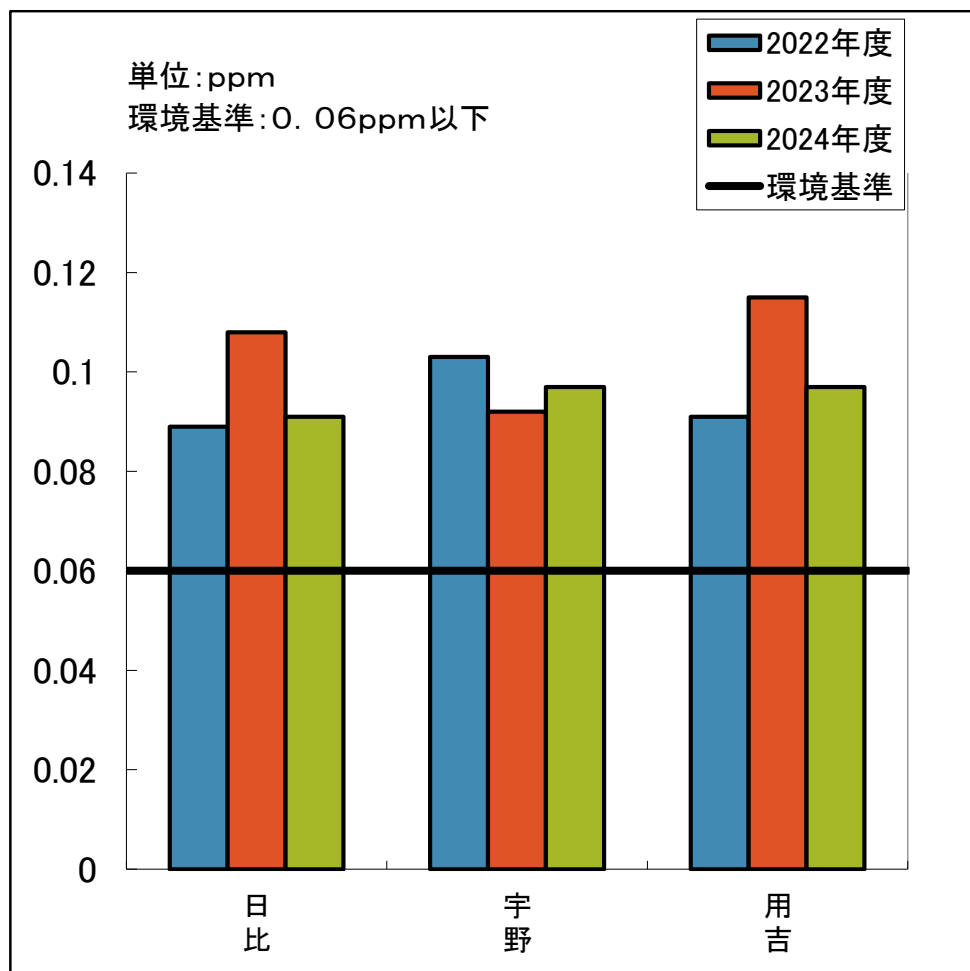
光化学オキシダント濃度の昼間1時間値の最高値
